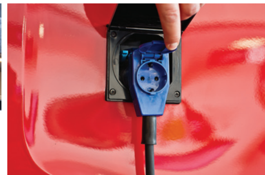
Externe CEE-Steckdose (für SHORT links, für LONG rechts) mit Möglichkeit einer 230V-Steckdose unter der Markise
